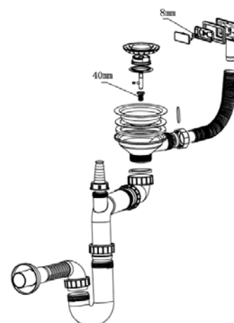
ВЫПУСК С СИФОНОМ ДЛЯ КОМПЗИТНОЙ КУХОННОЙ МОЙКИ с отводом для стиральной машины и гибкой трубой Перелив БОКОВОЙ Прямоугольный с планкой Диаметр выпуска 90 мм. Резьба 40 мм СТАЛЬ
