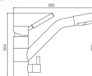
Смеситель трёхканальный
