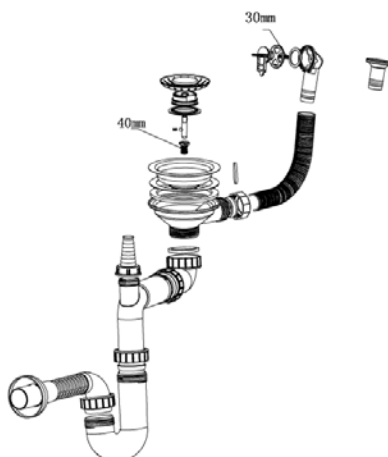
ВЫПУСК С СИФОНОМ ДЛЯ КОМПЗИТНОЙ КУХОННОЙ МОЙКИ с отводом для стиральной машины и гибкой трубой Перелив БОКОВОЙ и ВЕРХНИЙ Круглый Диаметр выпуска 90 мм. Резьба 40 мм СТАЛЬ
