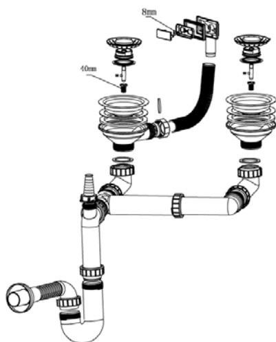
ВЫПУСК ДВОЙНОЙ С СИФОНОМ ДЛЯ КОМПЗИТНОЙ КУХОННОЙ МОЙКИ с отводом для стиральной машины и гибкой трубой Перелив БОКОВОЙ Прямоугольный с планкой Диаметр выпуска 90 мм. Резьба 40 мм СТАЛЬ
