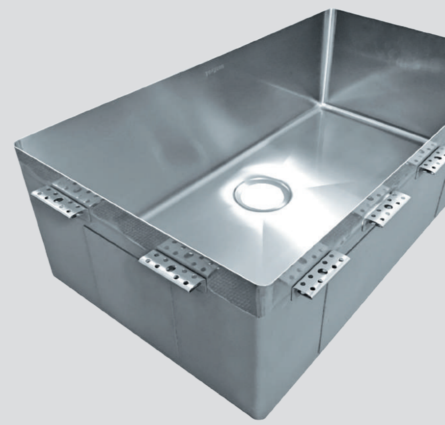
Новый метод монтажа TOPZERO
